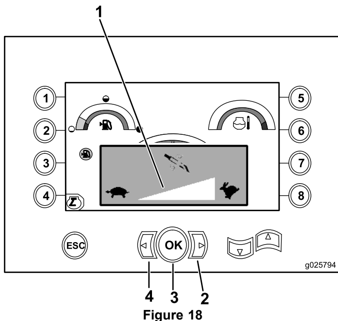
Écran de vitesse de rotation de forage
