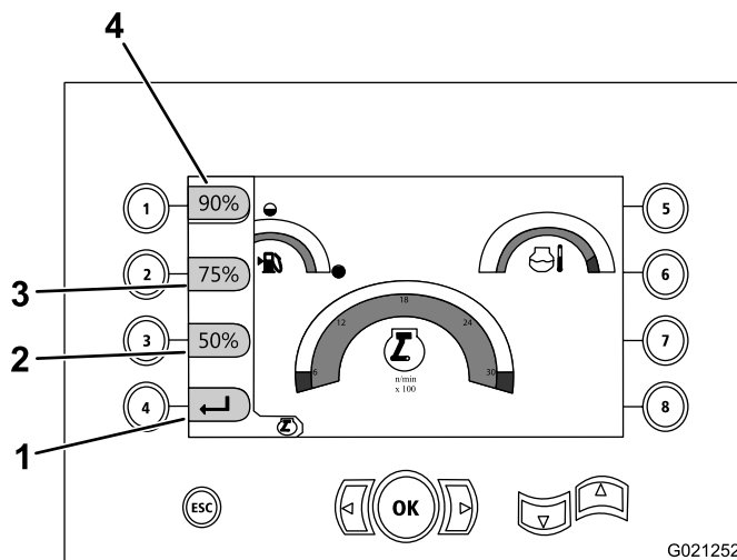
Écran de commande de puissance
