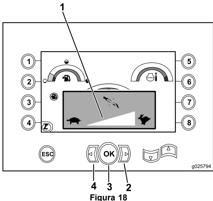
Tela de velocidade de giro da perfuratriz
