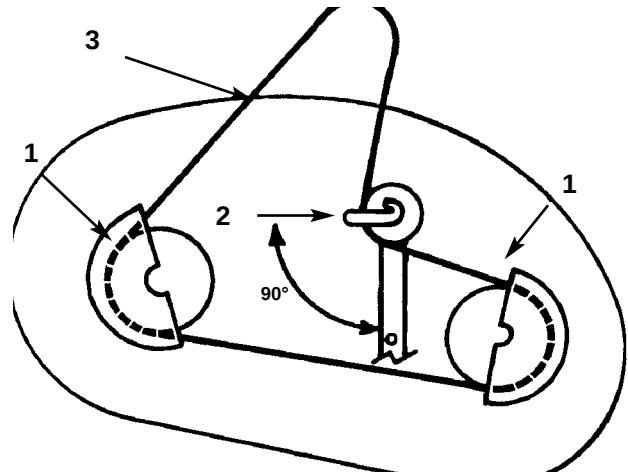
Figuur 48 Bovenaanzicht
