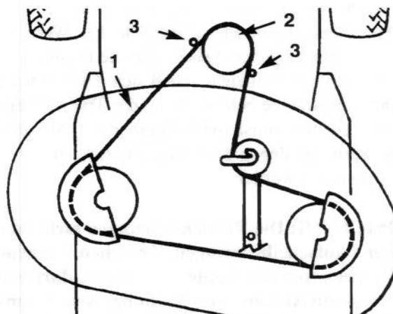
Bild 43 Obenansicht
