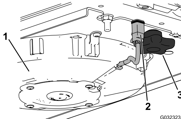
Figur 91 Höger fläkt visas
