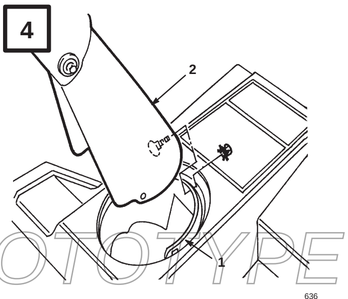
1. Utkastarring 2. Snöutkastare
