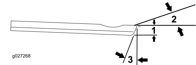
图28 建议的顶面和前底刀研磨角度
