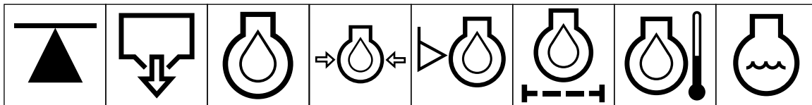
Macaco ou ponto de apoio Drenagem/Escoamento Óleo de lubrificação do motor Pressão do óleo de lubrificação do motor Nivel do óleo de lubrificação do motor Filtro do óleo de lubrificação do motor Temperatura do óleo de lubrificação do motor Líquido de refrigeração do motor
