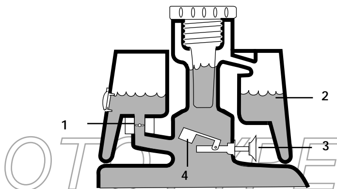
Figura 10 FUNCIONAMIENTO NORMAL (aceite caliente)
