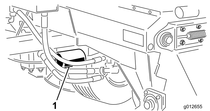
1. 液压油滤芯
