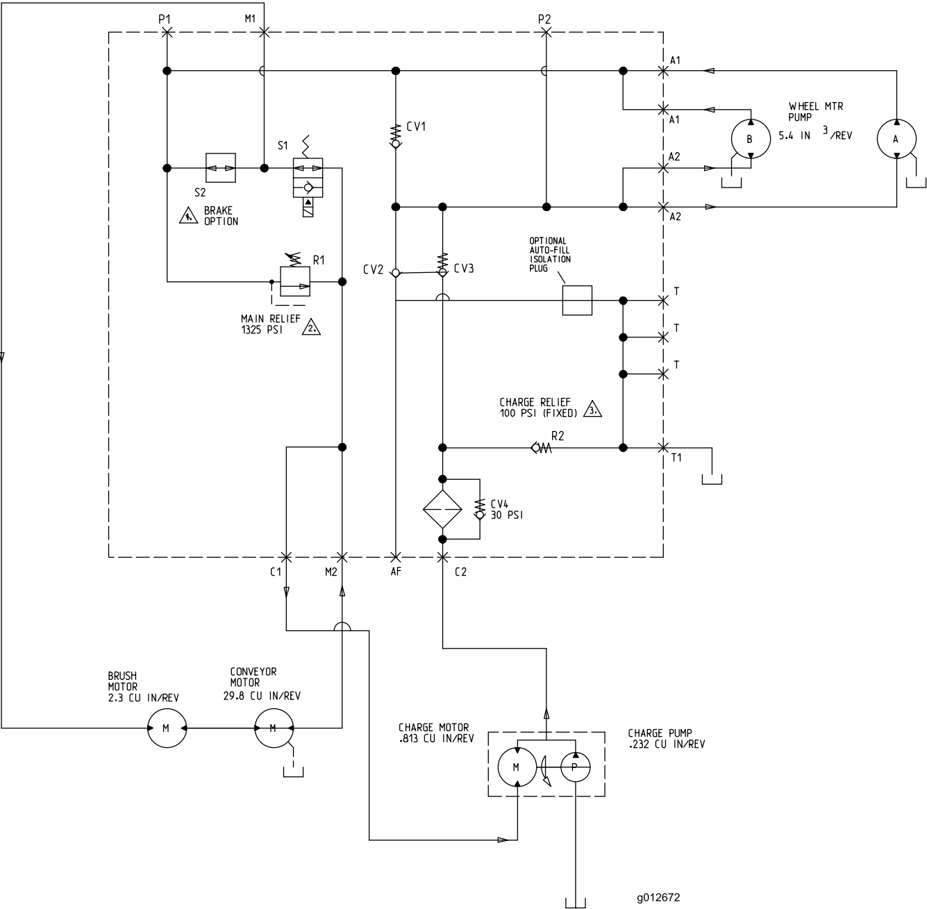
液压系统示意图 (Rev. 1)
