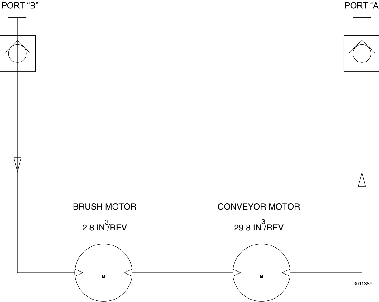
液压系统示意图 (Rev. A)
