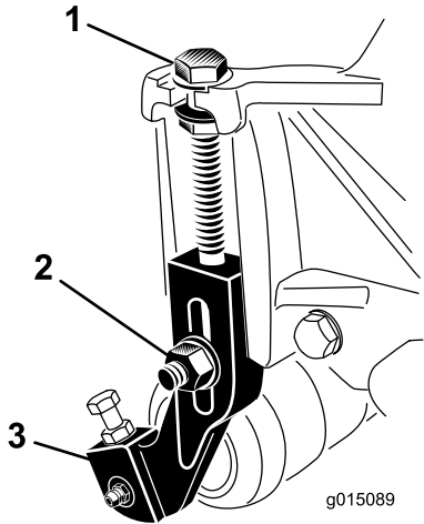
图18 图中为 8 刀片滚刀组
