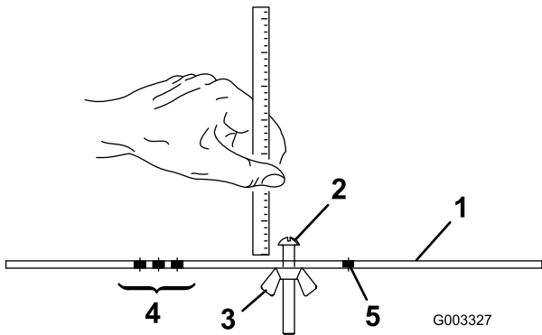
图19 1. 调刀尺 2. 高度调节螺丝 3. 螺母 4. 用于设置疏草刀疏草高度的孔 5. 未使用的孔
