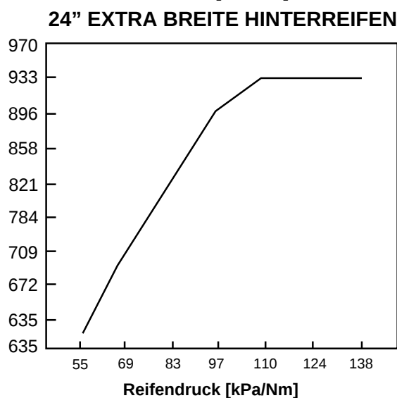
Maximale Gesamtbelastung der Hinterachse
