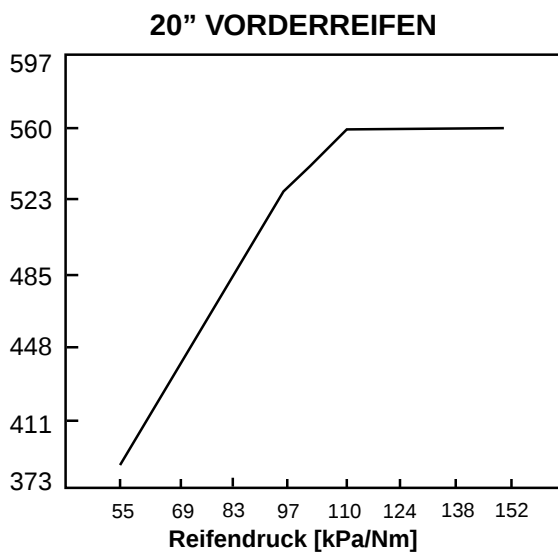
Maximale Gesamtbelastung der Vorderachse
