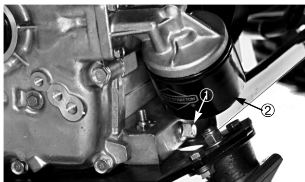
Fig. 15 1. Dreneringsplugg 2. Oljefilter
