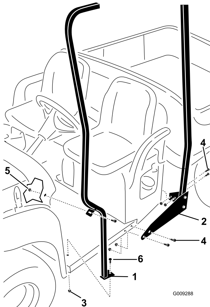
Figuur 3 Linkerkant getoond
