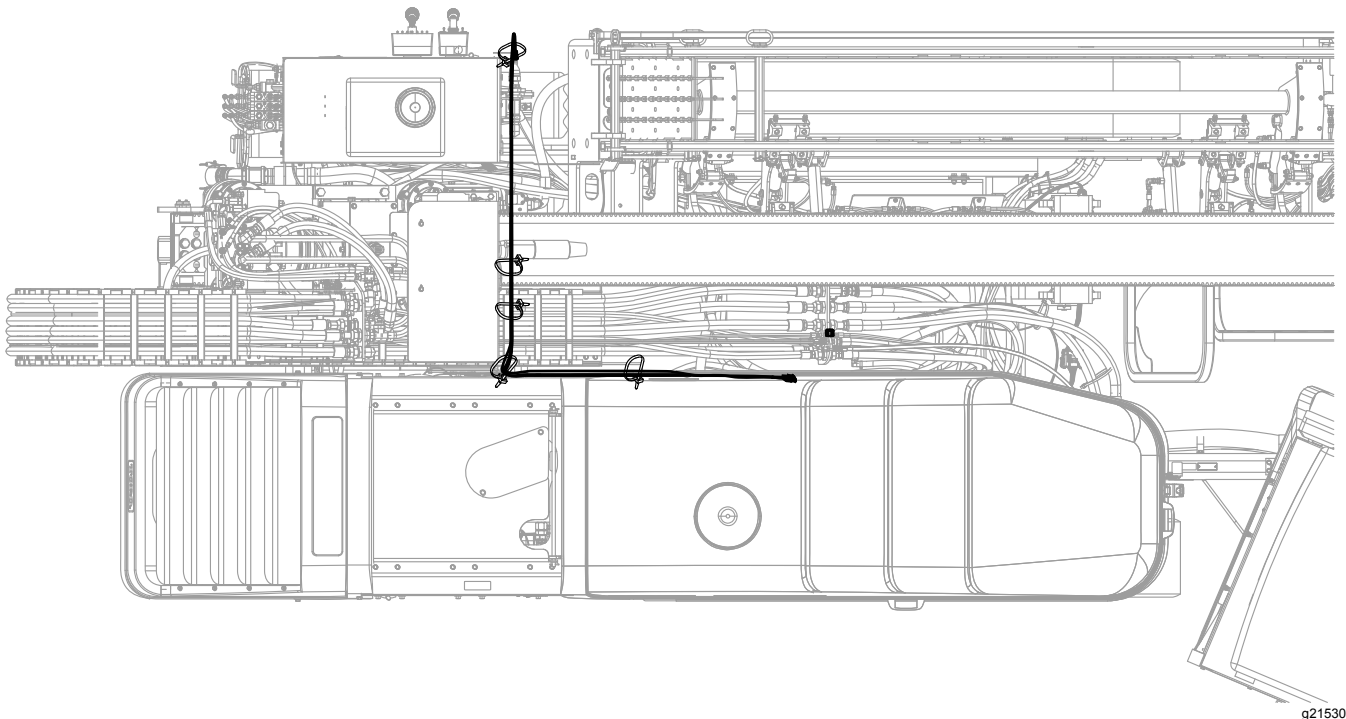
Figur 7 Kablageöversikt
