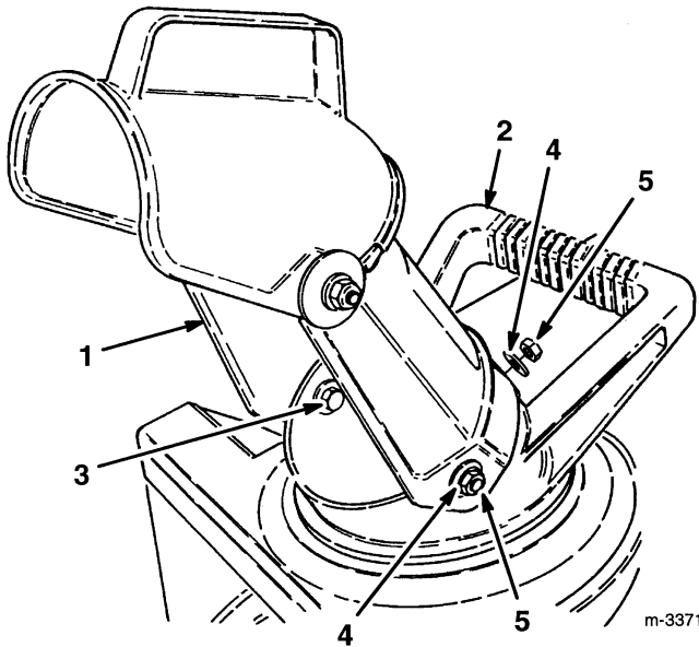
1. Auswurfkanal 2. Auswurfkanalgriff 3. Sechskantschraube 4. Unterlegscheibe 5. Sicherungsmutter
