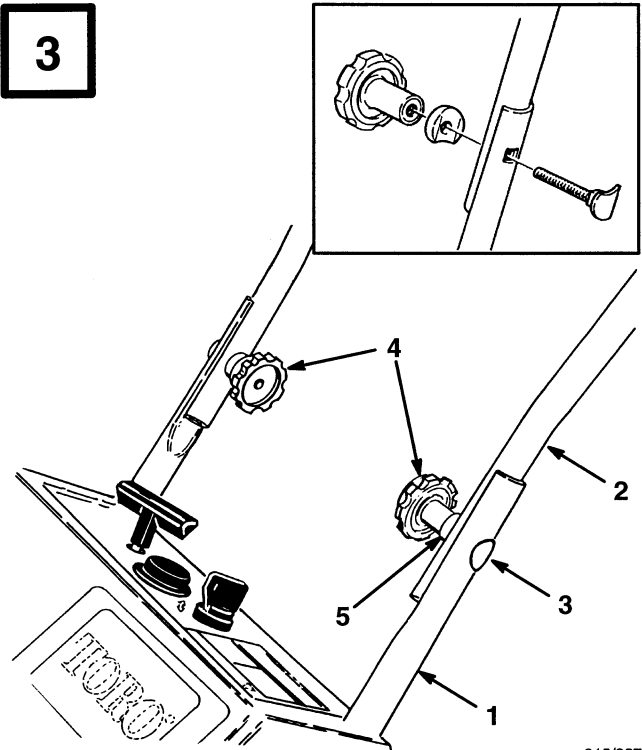
1. Unterer Griffholm 2. Oberer Griffbügel 3. Linsenkopfschraube 4. Knopf 5. Gekrümmte Unterlegscheiben
