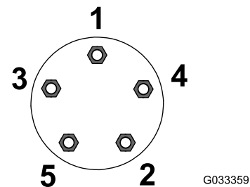
Figura 16 Ruedas traseras
