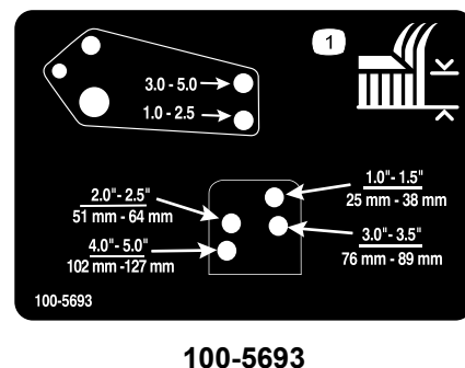
1. Schnitthöheneinstellung
