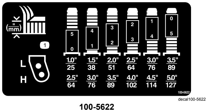
1. Schnitthöheneinstellung
