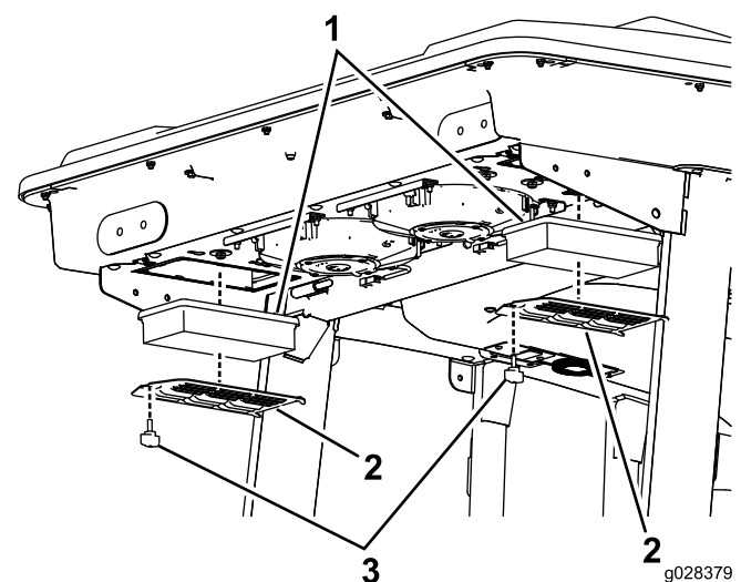
Figur 116 Lufffilter bakom hytten
