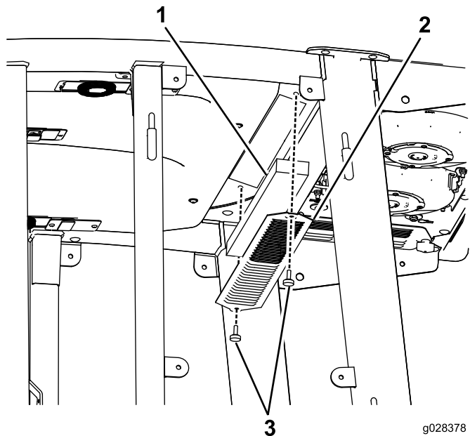
Figur 115 Lufffilter i hytten
