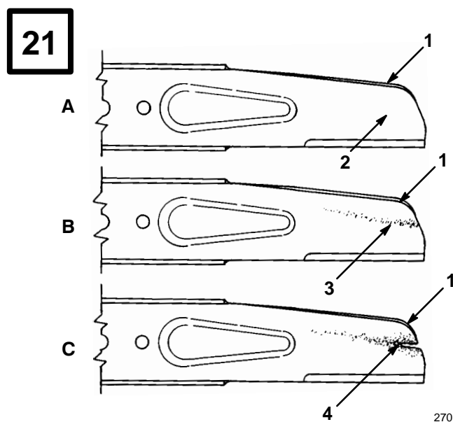
1. Partie incurvée 2. Partie plane de la lame 3. Usure 4. Formation d'une entaille
