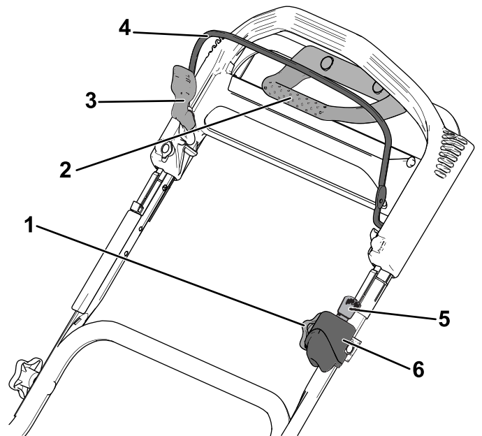
Bild 10 Oberer Holm
