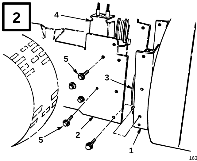
1. Walzengehäuse 4. Führungsrolleneinheit 2. Motorrahmen 5. Befestigungsschrauben (2) 3. Gebläserad- Riemenscheibe
