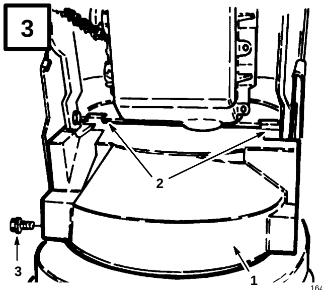
1. Nederste remdeksel (vist fra bunnen) 2. Monteringsflenser 3. Flenshodeskrue
