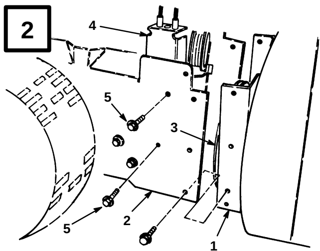
1. Spiralbladhus 2. Motorramme 3. Remskive for viftehjøl 4. Lederull-enhet 5. Monteringsskruer (2)
