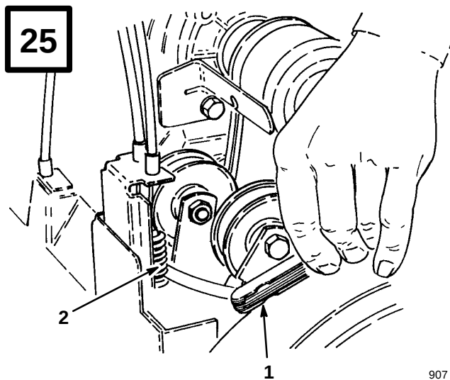
1. Følelære
