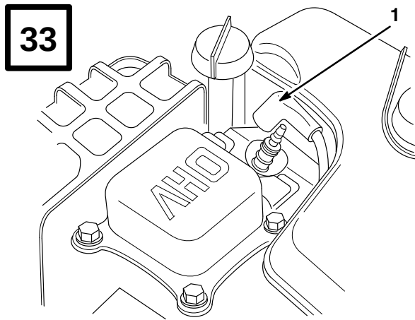
1. Tennpluggkabel
