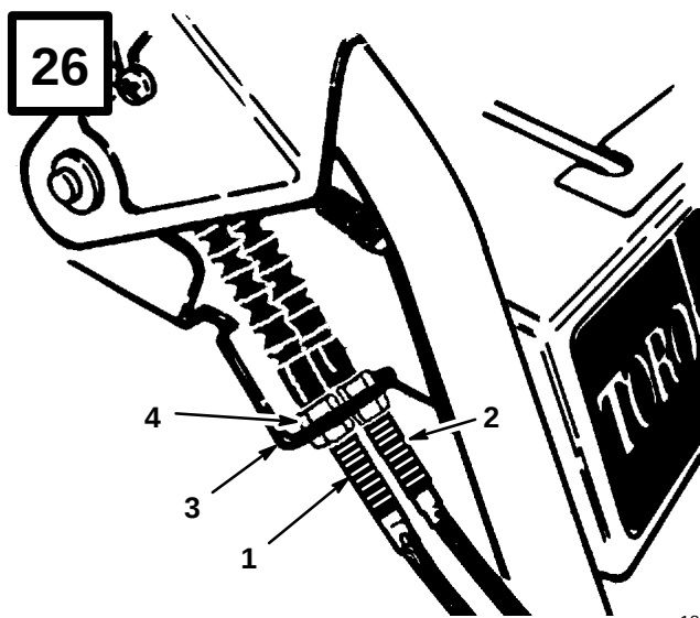
1. Kabel for spiralblad/ viftejul (ytterste kabel) 2. Trekk-kabel (innerste kabel)
