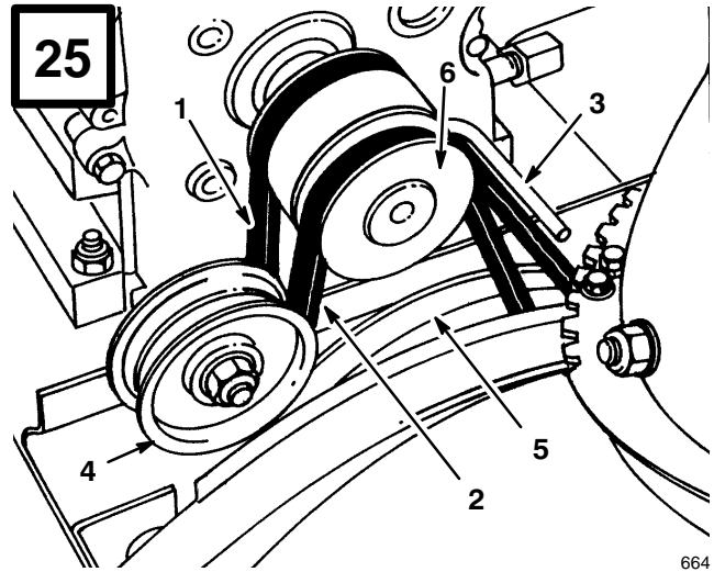
1. Cinghia di trazione della trazione 2. Cinghia di trazione di coclea/ventola 3. Guida della cinghia 4. Puleggia tendicinghia 5. Puleggia grande di coclea/ventola 6. Puleggia del motore
