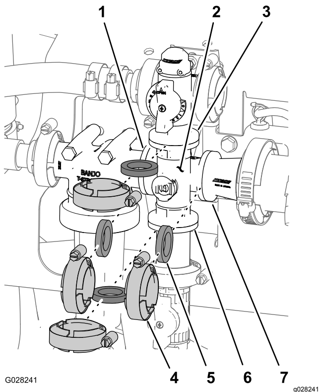
Figure 78 Vanne d'agitation
