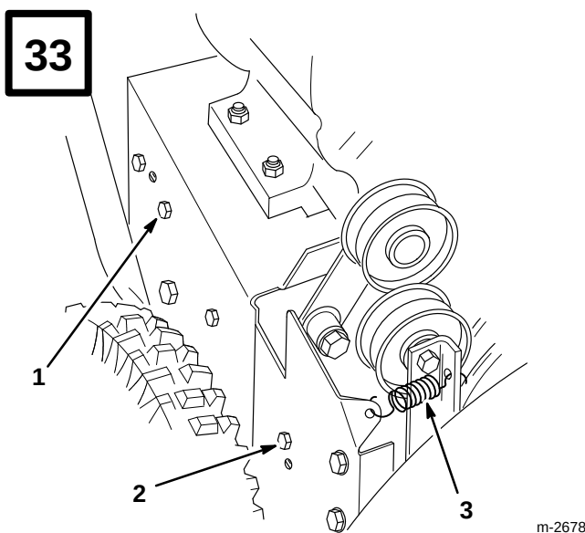
1. Bakre skruv
