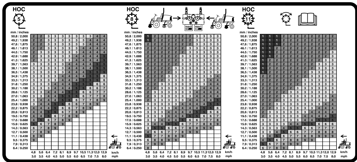
그림31 127mm 릭 속도 차트
