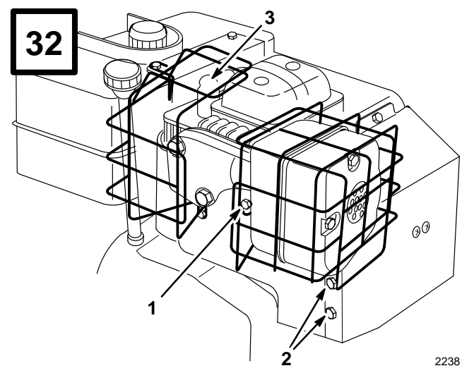
1. Skrue - eksospotteskydd (1) 3. Tennpluggkabel 2. Skrue med sekskanthode (2)
