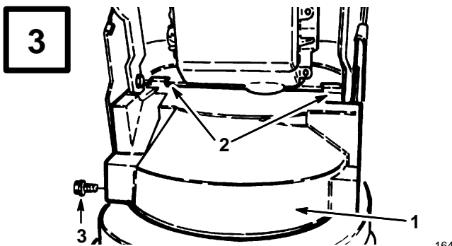
1. Nederste remdeksel (vist fra bunnen) 2. Monteringsflenser 3. Flenshodeskrue
