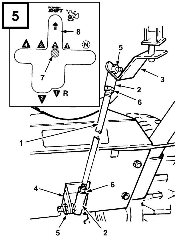
1. Girstag 2. Kuleledd 3. Girbrakett 4. Transmisjonsspak 5. Kontramutter 6. Sikringsmutter 7. Girvekslingsspak 8. "Power Shift"-spor
