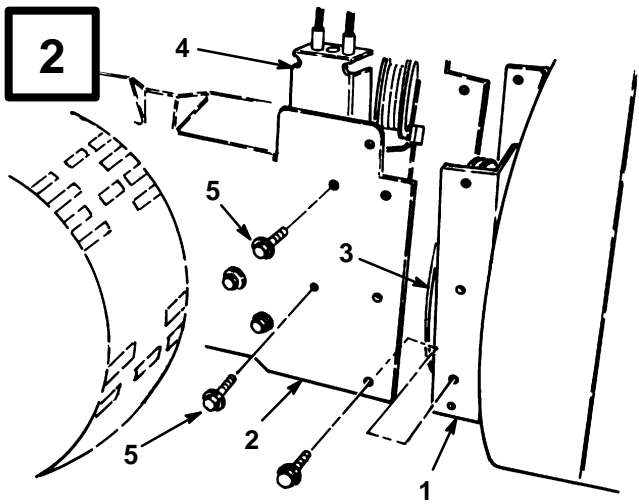
1. Spiralbladhus 2. Motorramme 3. Remskive for viftehjul 4. Lederull-enhet 5. Monteringsskrue (2)
