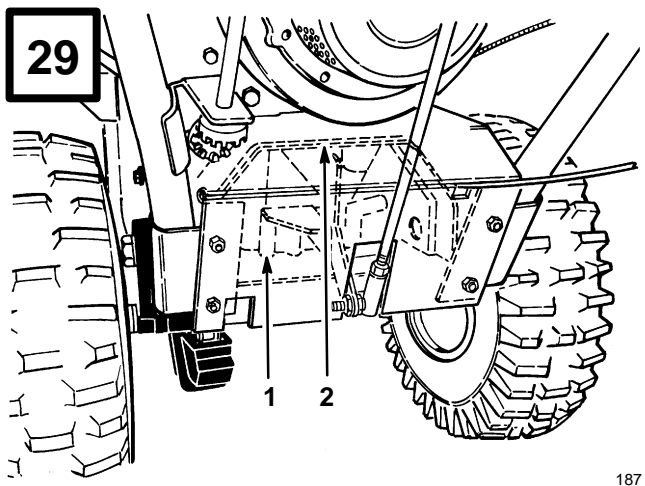
1. Transmisjon 2. Transmisjonsramme
