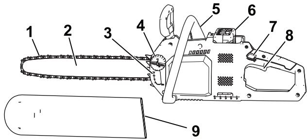
Figure 4 Côté gauche de la tronçonneuse
