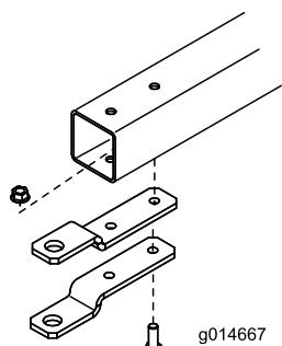
图7 低挂钩位置
