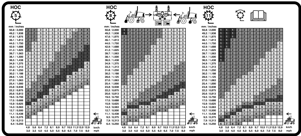
Figura 70 Tabella della velocità dei cilindri 177,8 mm
