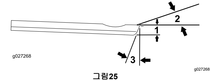
상단 및 전면 베드나이프 권장 연마 각도(그림25)
