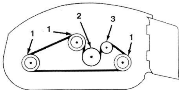
Bild 12—Riemenlauf
