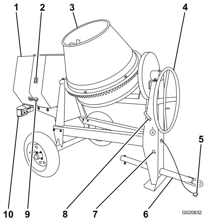
Figura 10 Modelos 68004C, 68006C, y 68009C
