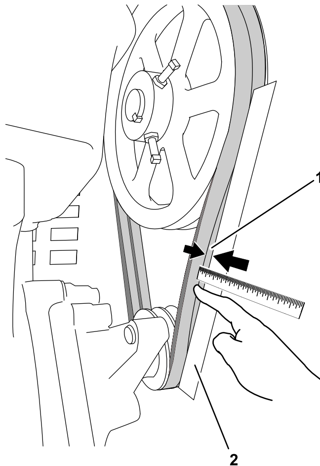
Figura 54 Correas de transmisión
