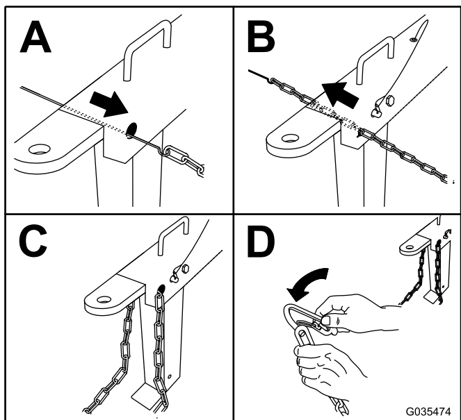
Figura 9 Modelos de descarga frontal
