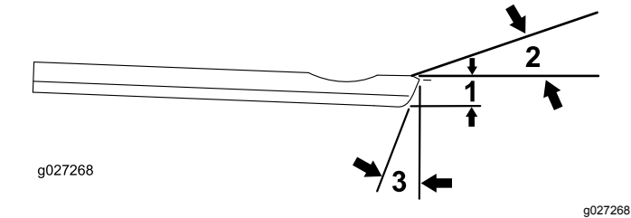
图27 建议的顶面和前底刀研磨角度
