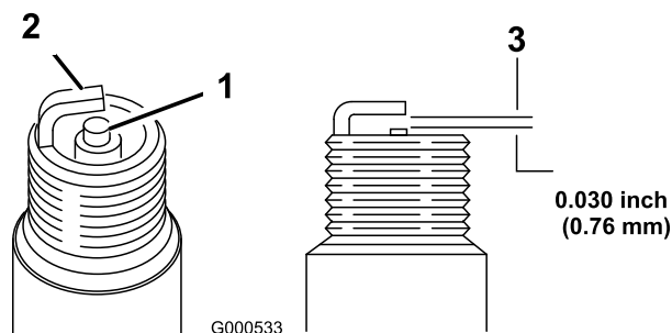
1. Mittelelektrodisisolator 2. Sidoelektrod 3. Luftgap (ej skalenligt)
