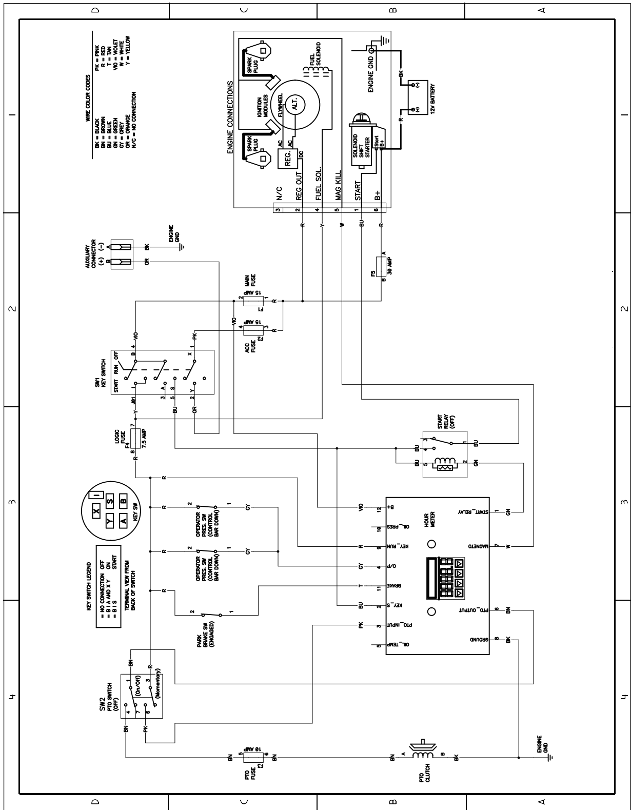
Esquema elétrico DWG 131-1199 (Rev. A)
