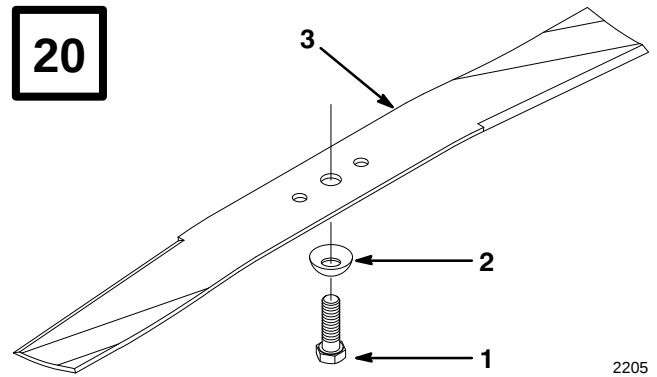
1. Schnittmesserschraube 2. Unterlegscheibe 3. Schnittmesser
