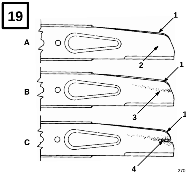
1. Segel 2. Flachseite des Schnittmessers 3. Verschleiß 4. Riefenbildung
