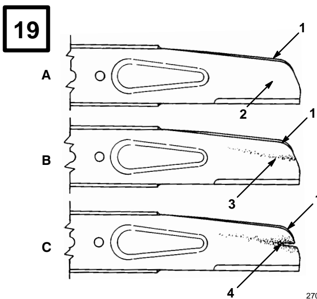
1. Alettatura 2. Parte piatta della lama
