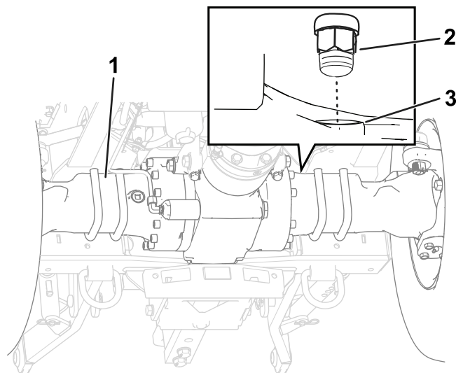
Figura 102 Assale posteriore
