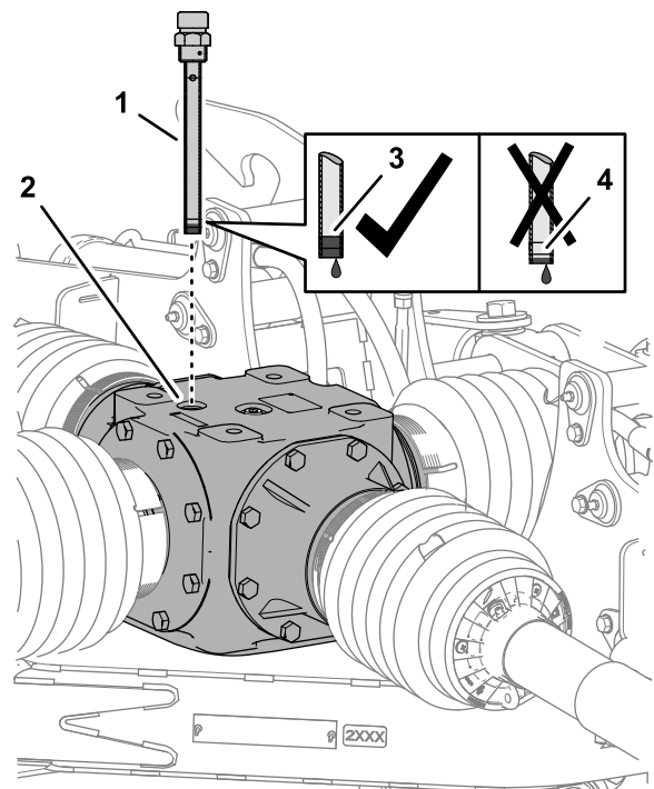
Figur 57 Mittväxellåda
