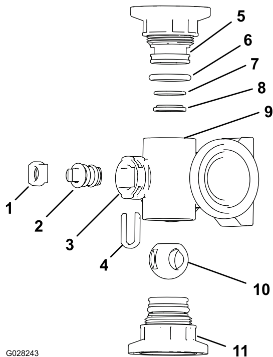
Figuur 114 Mengklepverdeler
