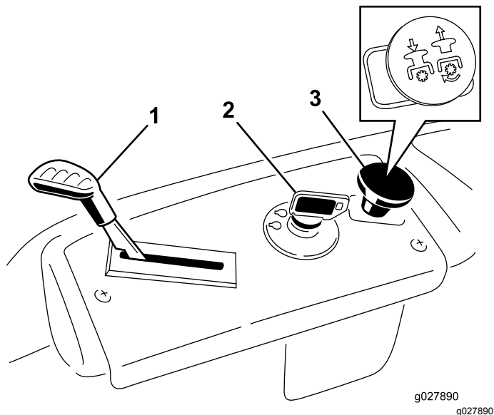
Рисунок 6 Панель управления
