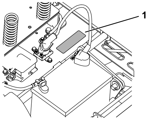
Рисунок 1 Под сиденьем
