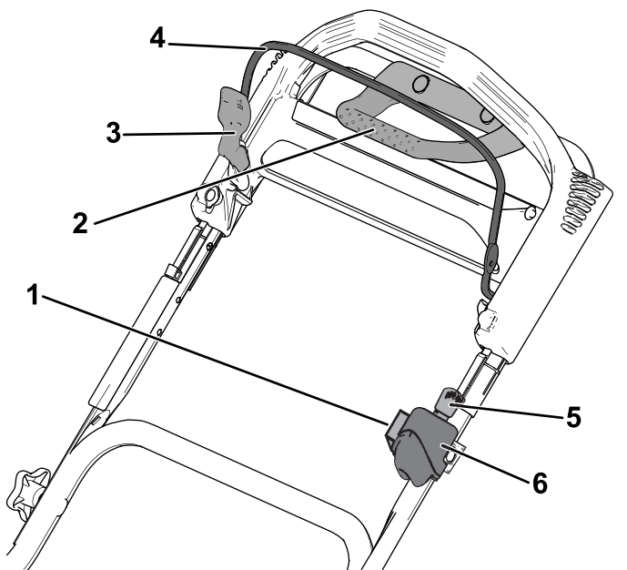
Figura 8 Manillar superior
