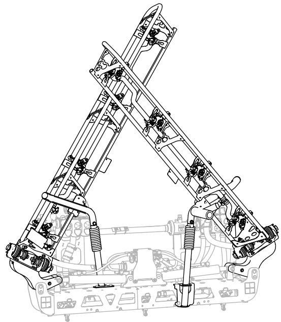
Kuva 43 X-kuljetusasento
