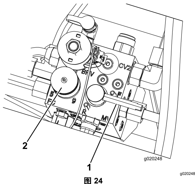
1. 倒磨控制杆
