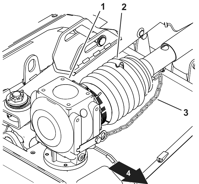
Figur 21 Högerklippdäckets drivaxelskydd
